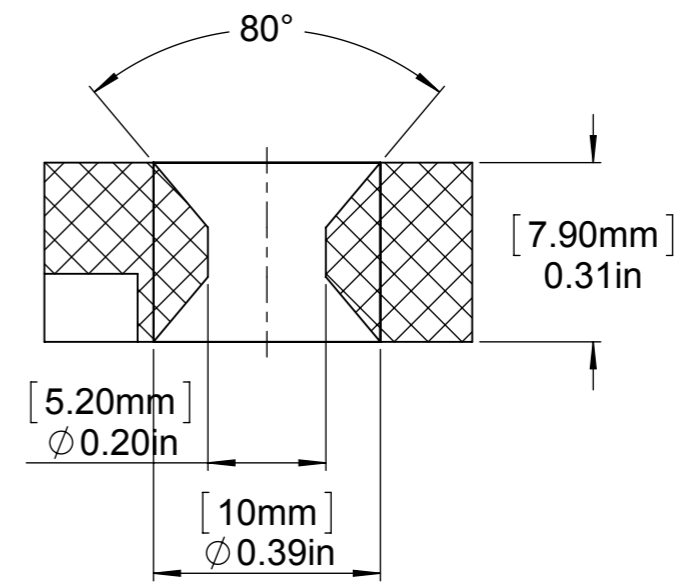
SECTION A-A SCALE 3 : 1
