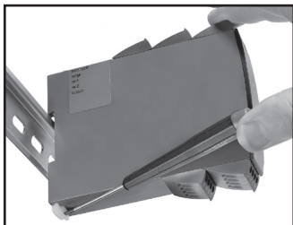
Figure 1 : Débloquez le verrou inférieur pour dégager le dispositif du rail DIN.
