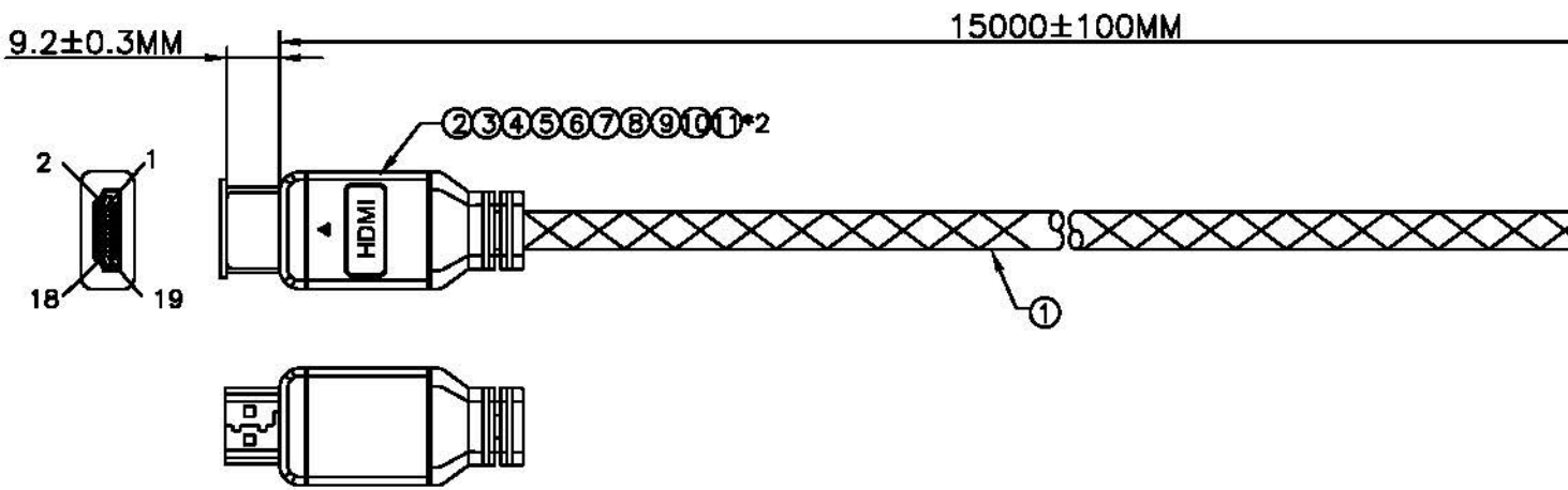
Conn.1 HDMI A Type Male
