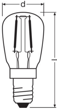
P SPC.T26 12 1.3 W/827 E14
