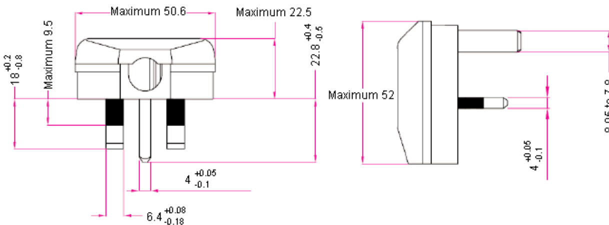
Dimensions : Millimetres
