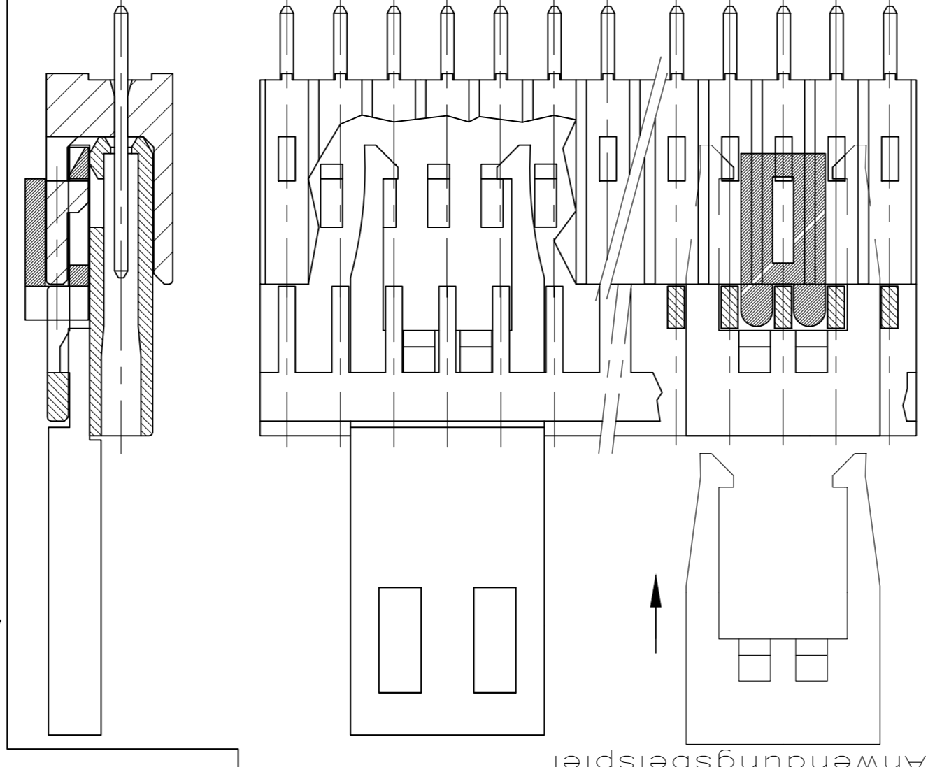
ASSEMBLED COMPONENTS (FOR EXAMPLE) Anwendungsbispiel
