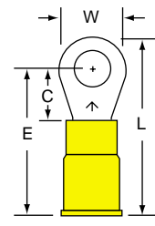
MVU10-10R Stud Size: 10 Wire Range: 12-10
