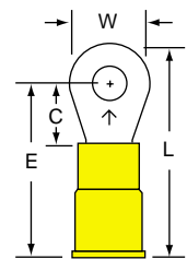
MVU10-8R Stud Size: 8 Wire Range: 12-10
