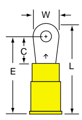
MVU10-4R/S Stud Size: 4 Wire Range: 12-10
