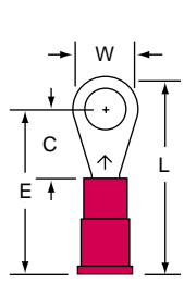
MVU18-10R/L Stud Size: 10 Wire Range: 22-18
