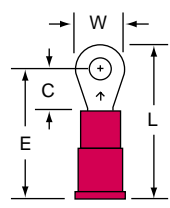
MVU18-4R/S Stud Size: 4 Wire Range: 22-18
