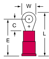
MVU18-6R/S Stud Size: 6 Wire Range: 22-18
