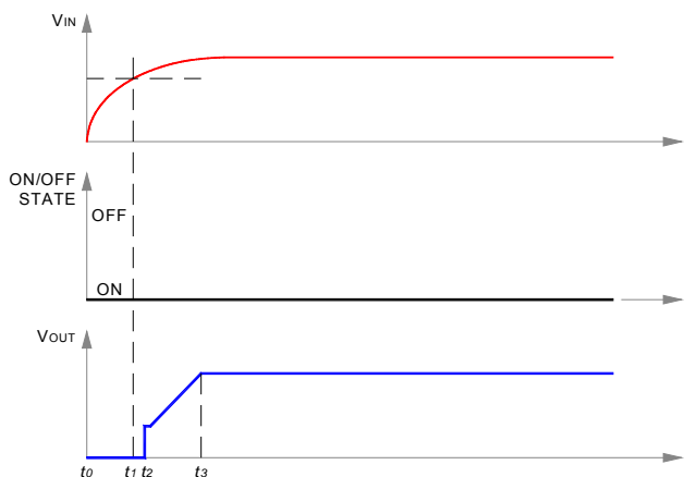
Fig. F: Startup scenario #1.
