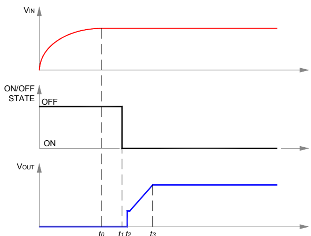
Fig. G: Startup scenario #2.
