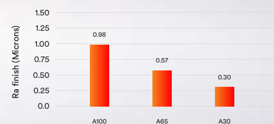
Ra finish – Trizact™ CF
