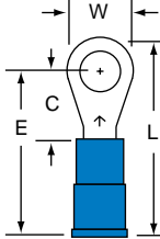
MNG14-10R/L Stud Size 10 Wire Range 16-14
