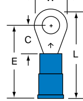
MNG14-8R Stud Size 8 Wire Range 16-14
