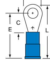
MNG14-8R/L Stud Size 8 Wire Range 16-14
