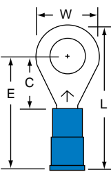
MNG14-14R/S Stud Size 1/4 Wire Range 16-14
