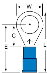
MNG14-516R/S Stud Size 5/16 Wire Range 16-14
