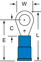
MNG14-10R Stud Size 10 Wire Range 16-14
