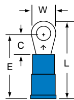
MNG14-6R/S Stud Size 6 Wire Range 16-14
