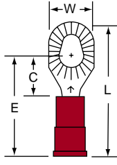
MNG18-610R Stud Size 6/8/10 Wire Range 22-18
