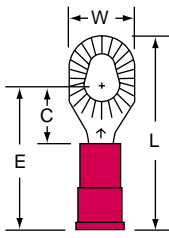
MV18-610R Stud Size 6/8/10 Wire Range 22-18
