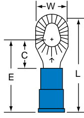
MNG14-610R Stud Size 6/8/10 Wire Range 16-14
