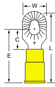
MNG10-610R Stud Size 6/8/10 Wire Range 12-10
