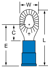
MV14-610R Stud Size 6/8/10 Wire Range 16-14
