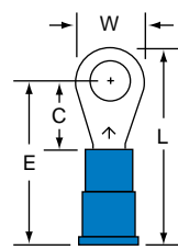
MV14-10R/L Stud Size 10 Wire Range 16-14
