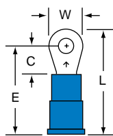
MVU14-4R/S
