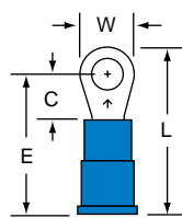
MVU14-6R/S
