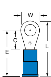
MVU14-10R/L
