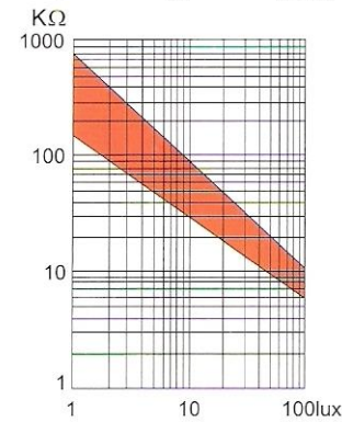
GL5549(GL5649)
