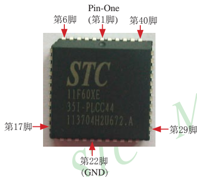
PLCC44封装实物图
