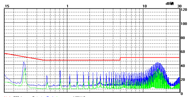
WRF1205S-3WR2 传导骚扰 Class B 测试效果图 (负线)
