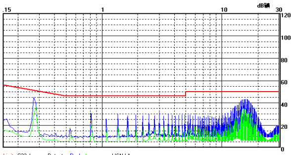
WRF1205S-3WR2 传导骚扰 Class B 测试效果图 (正线)
