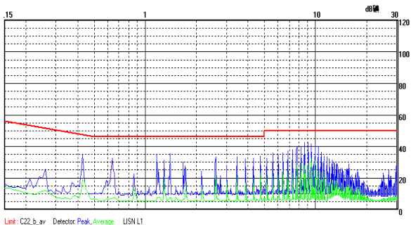
WRE2415S-3WR2 传导骚扰 Class B 测试效果图 (正线)
