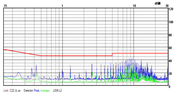
WRE2415S-3WR2 传导骚扰 Class B 测试效果图 (负线)
