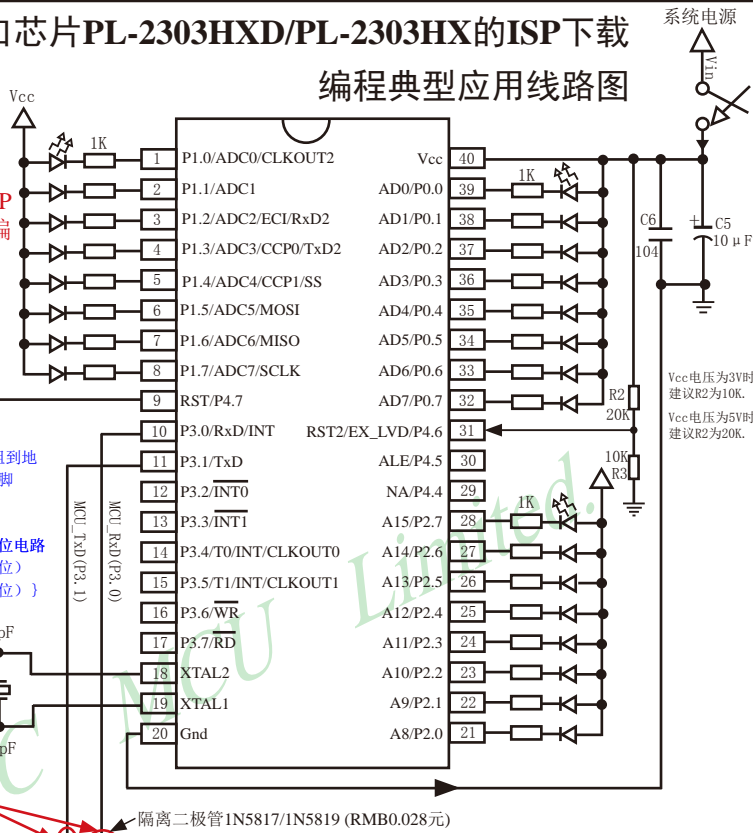
隔离二极管1N5817/1N5819 (RMB0.028元) STC 单片机在线编程线路 USB转串口
