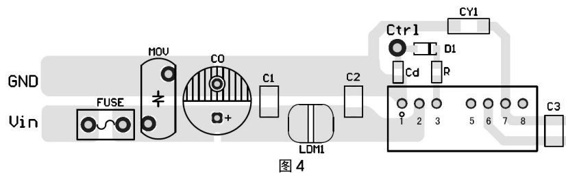
注: 输入输出地之间(CY)焊盘最小距离要保证≥2mm。
