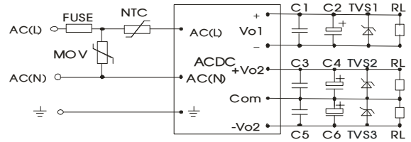
图 4: LH05-10Cxx(三路)系列典型应用电路
