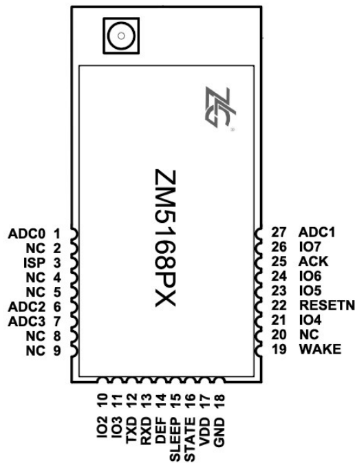
图 2.3 引脚分别图
