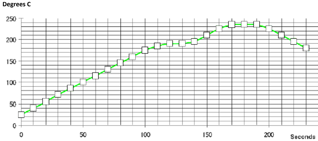
图表 2.1 推荐的回流焊温度曲线
