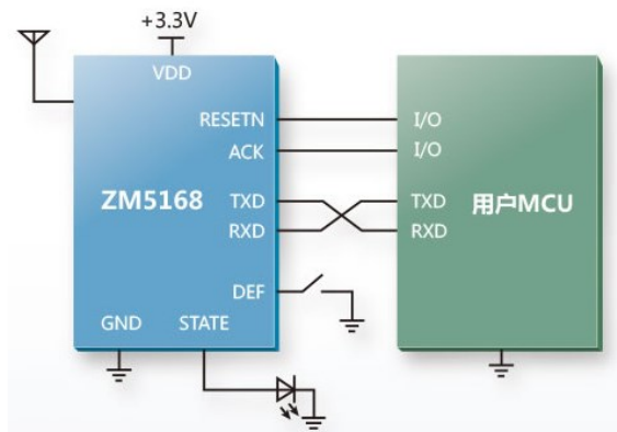
图 2.4 典型应用图
