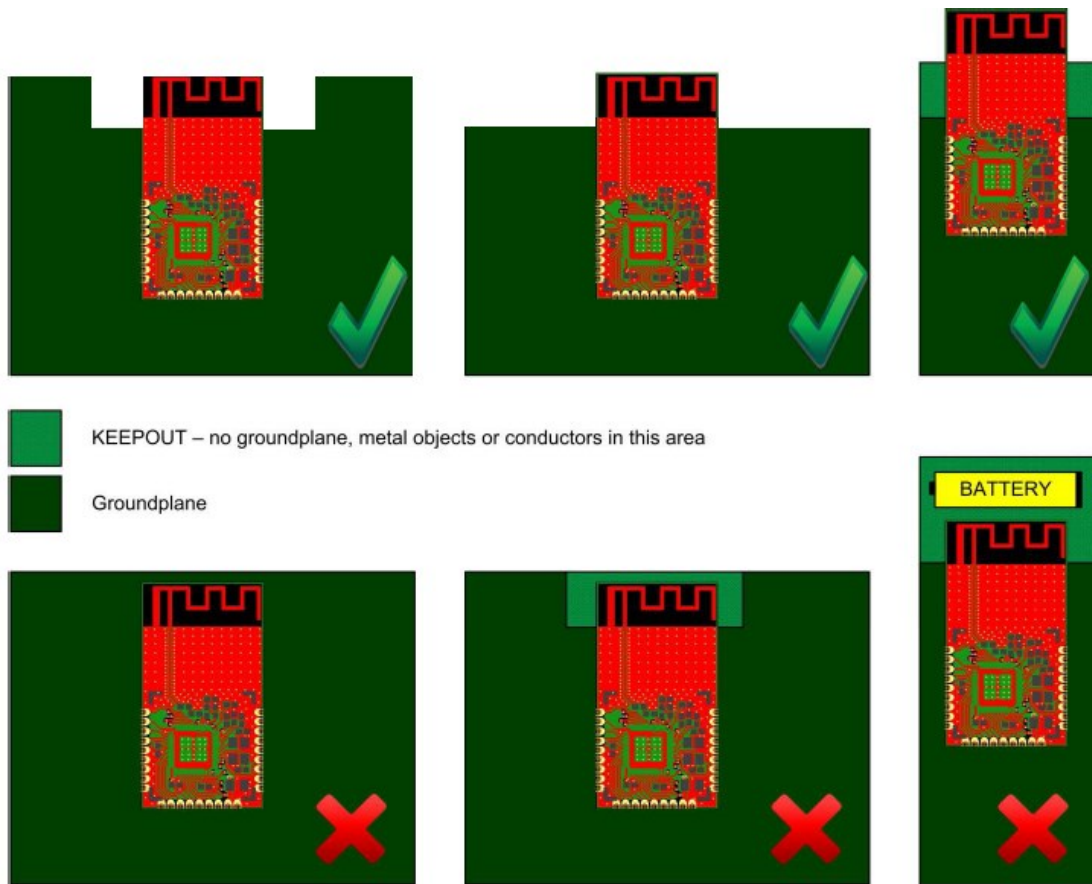
图 2.4 PCB 天线布局规范
