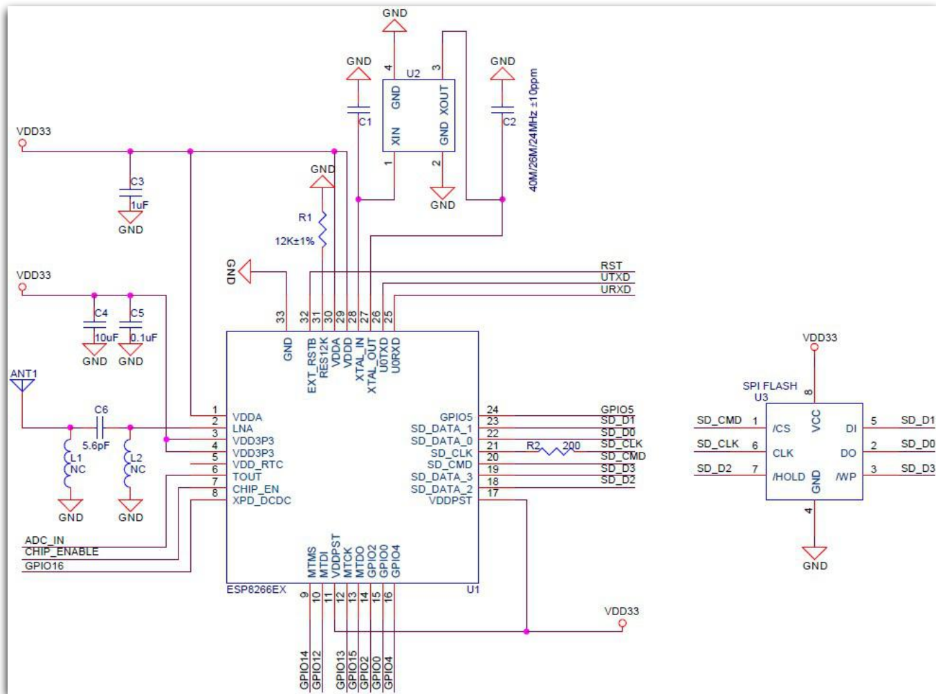
图 5 ESP-07 原理图
