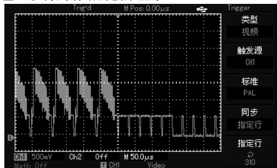
图3-9 视频行触发
