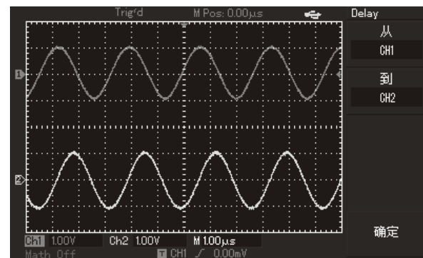
图3-2：波形延时
