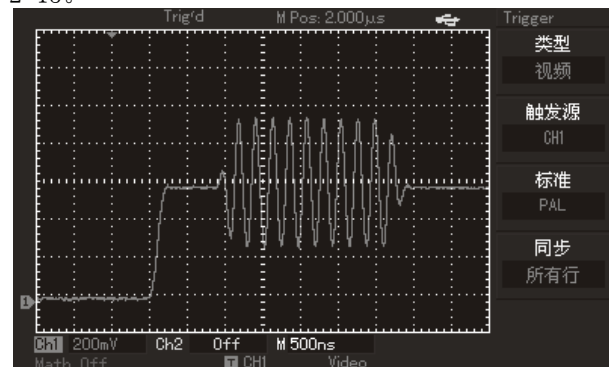
图2-14 视频触发：行同步
