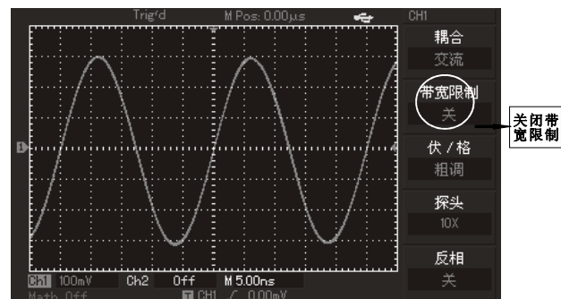
图2-4 带宽限制关闭时的波形显示
