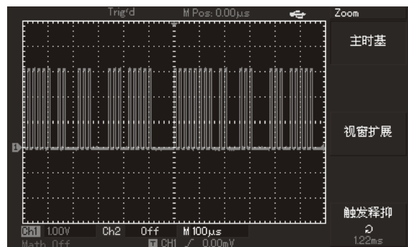
图2—17 触发释抑用以同步复杂波形
