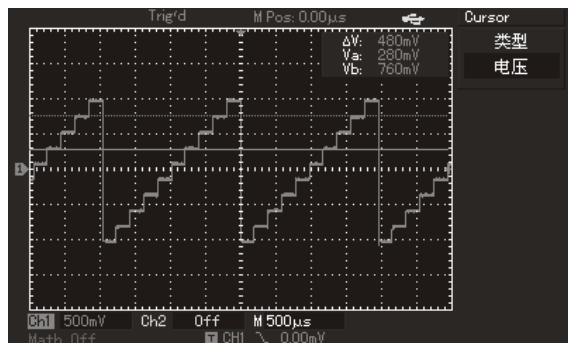
图3-6 光标测量信号电压差
