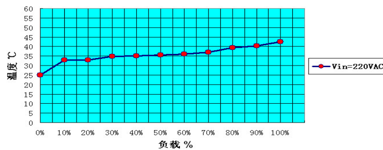
模块壳温曲线
