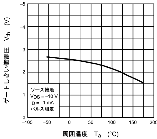
図 8.9 V_{th} - T_a (注8)
