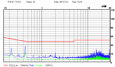
E2415S-2WR2 传导骚扰测试效果图 (负线)
