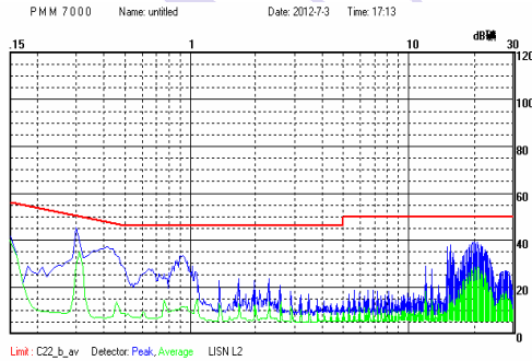
F2405S-2WR2 传导骚扰测试效果图 (负线)
