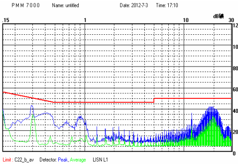
F2405S-2WR2 传导骚扰测试效果图 (正线)
