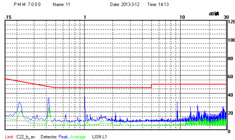
E2415S-2WR2 传导骚扰测试效果图 (正线)
