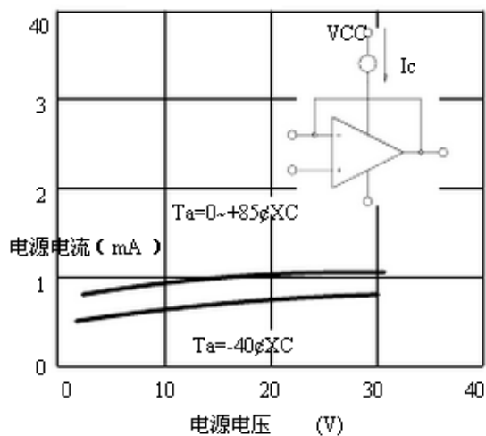
图 7-3. 电源电流
