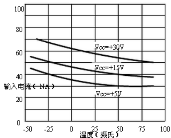
图 7-2. 输入电流
