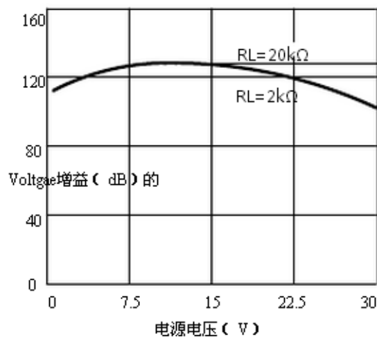
图 7-4 电压增益
