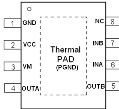
HSOP8
