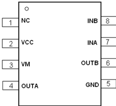
SOP8
