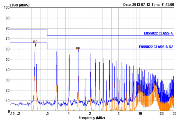
VD10-24S05B1 传导骚扰电源负极测试结果
