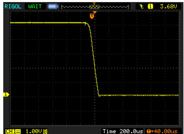
输出下降时间波形图 (标称满载)
