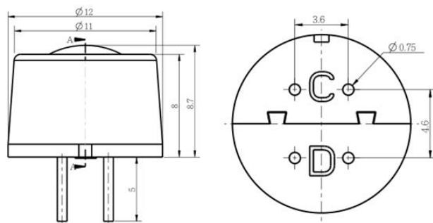
图 1: 元件外形结构
