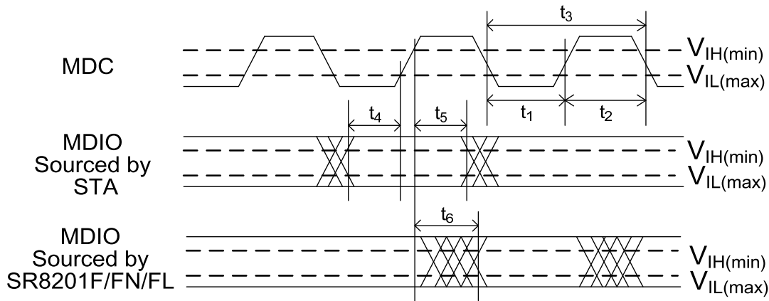
图 29.MDC/MDIO时序
