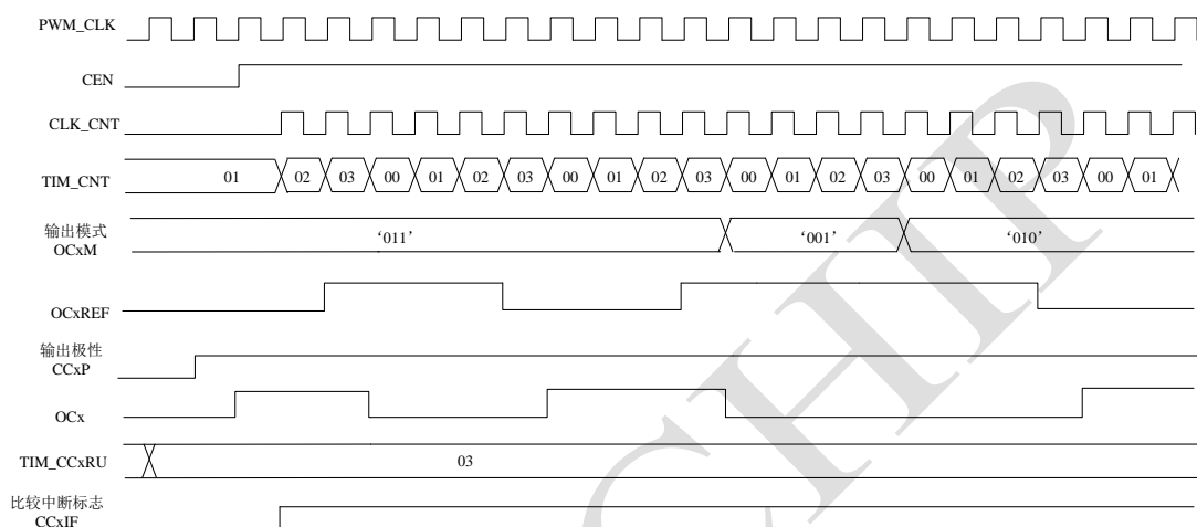
Figure 48 高级定时器比较输出模式
