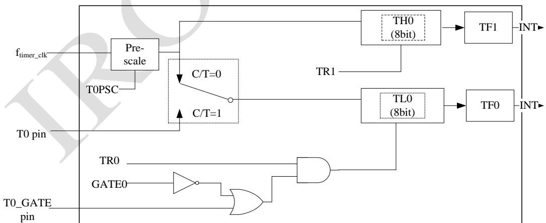
Figure 17 timer0 模式 3 实现框图
