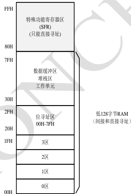
Figure 11 内部数据存储器分区
