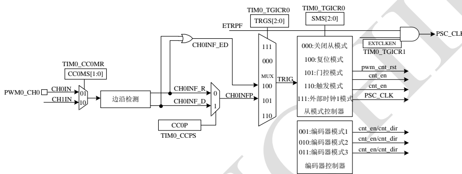
Figure 36 输入脚 PWM0_CH0 的信号作为外部时钟的连接例子
