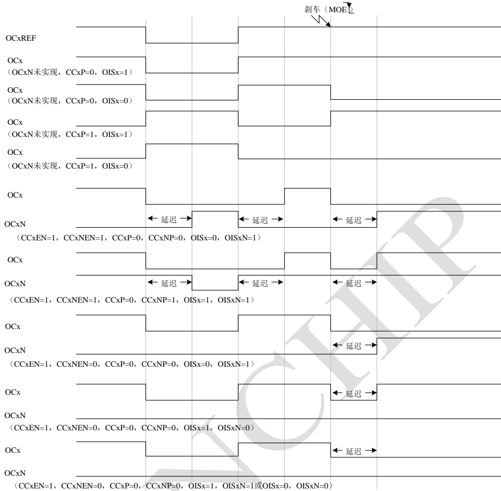
Figure 56 高级定时器刹车输出
