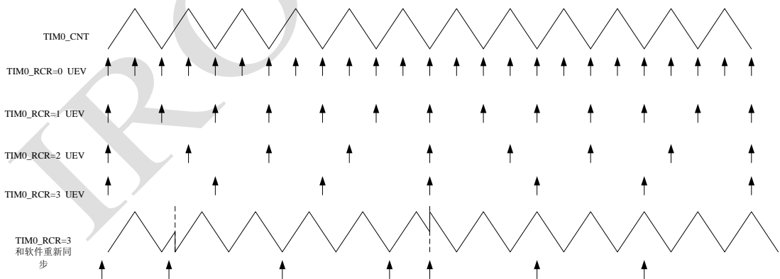
Figure 34 中央对齐计数模式下，重复计数次数分别为 0、1、2、3 时更新事件的产生
