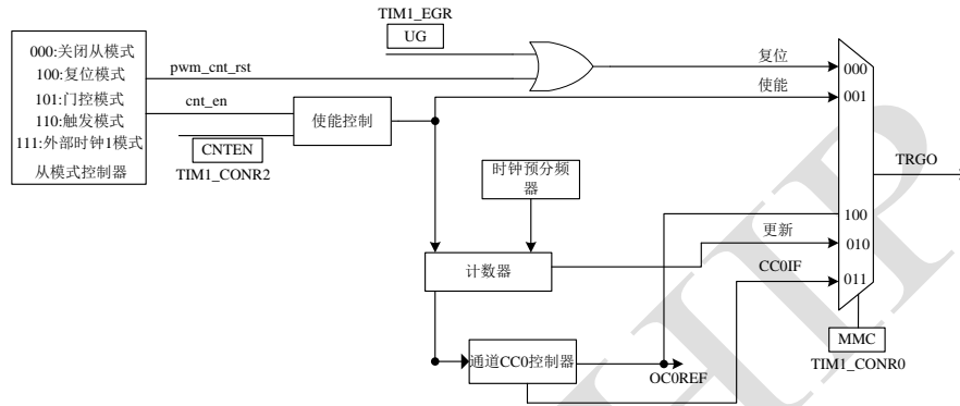
Figure 90 主模式控制示意图
