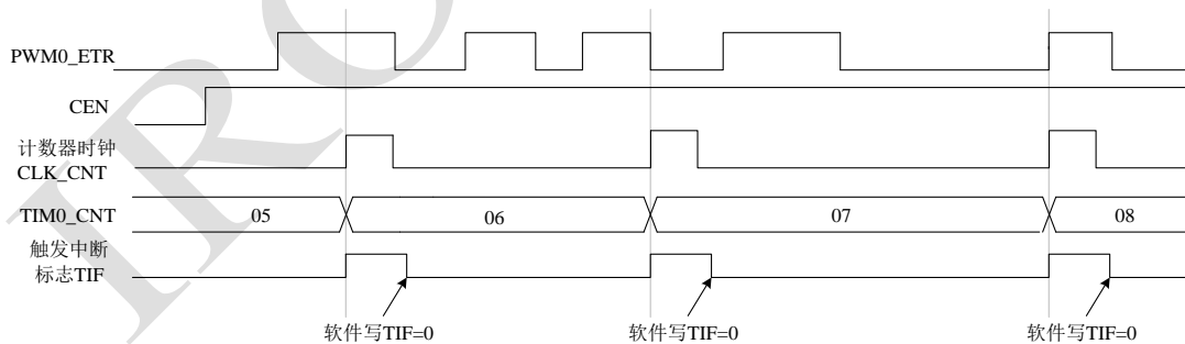
Figure 39 外部时钟模式 2 下计数器的时序图
