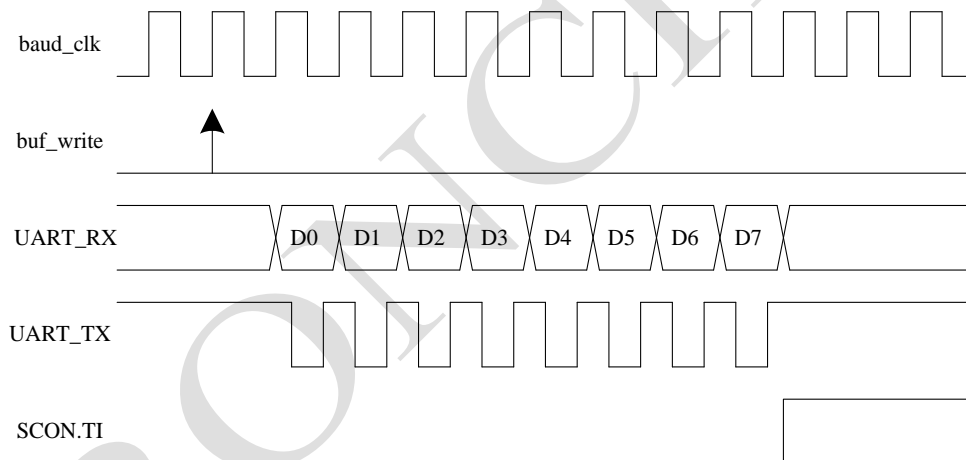
Figure 93 UART 模式 0 发送时序
