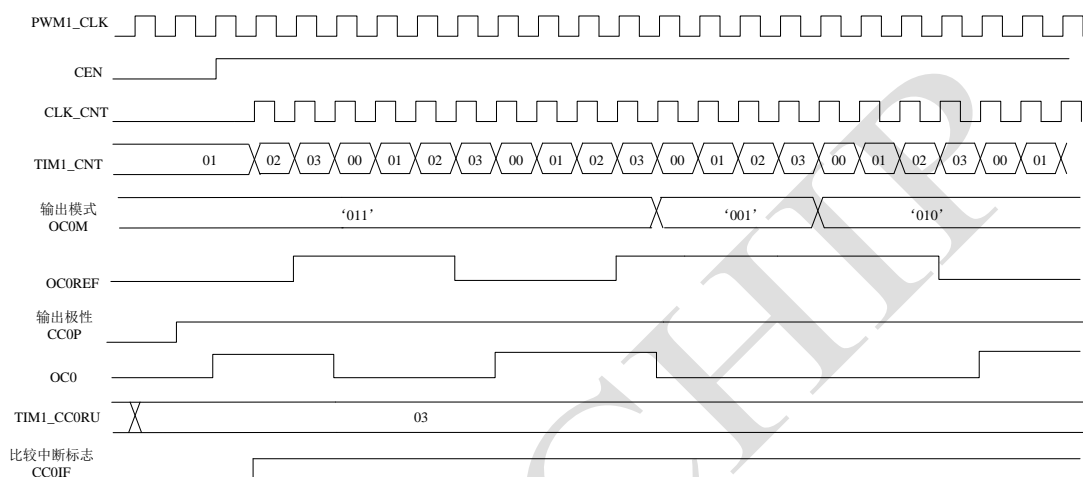
Figure 82 高级定时器比较输出模式
