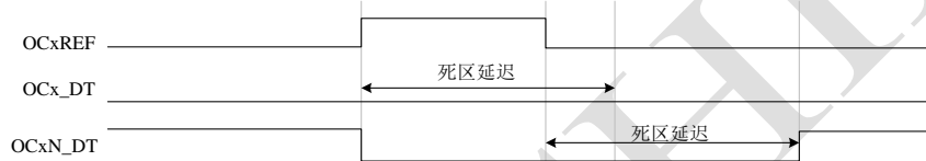
Figure 53 死区时间大于 OCxREF 无效电平宽度时的死区插入
