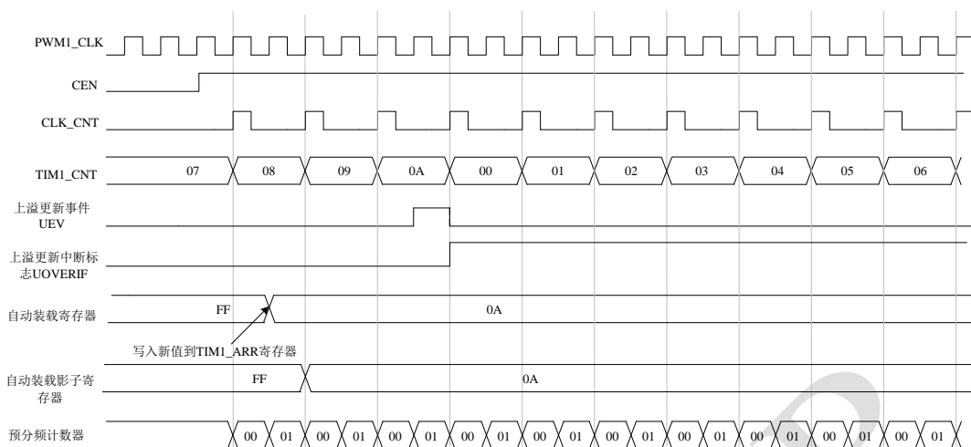
Figure 65 向上计数模式下，当自动装载寄存器的预装载功能不使能时计数器的时序图
