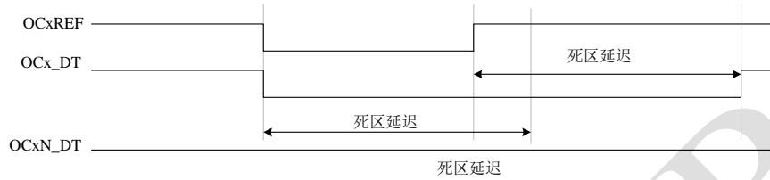
Figure 52 正常死区插入
