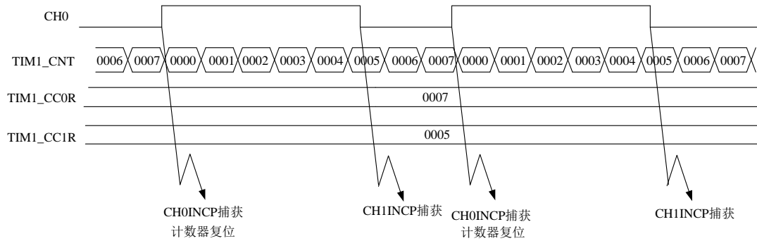
Figure 79 PWM 输入模式时序图
