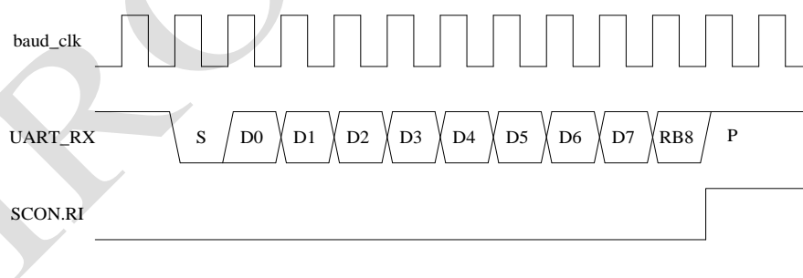
Figure 98 UART 模式 2 接收时序
