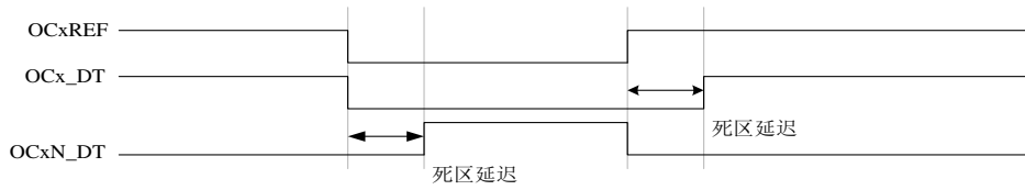
Figure 52 正常死区插入
