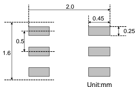
VTDFN1.6x1.6-6
