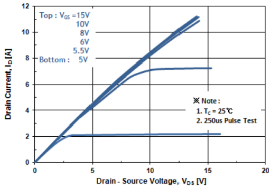
Fig. 1 I_D - V_{DS}
