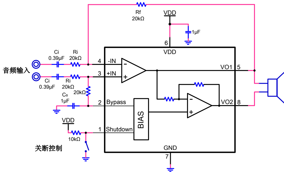
图 3. LM4871 差分输入模式电路图
