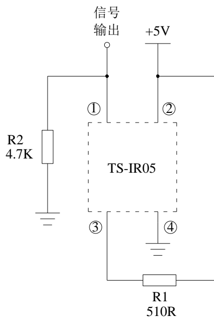
DC 5V 典型應用電路
