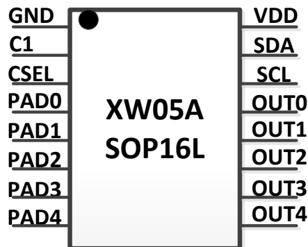
芯片引脚图
