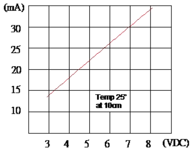
mA-V
