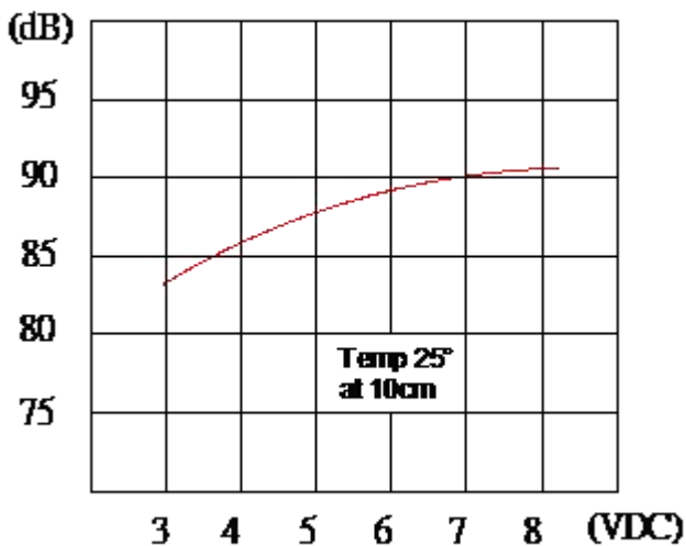
dB-V
