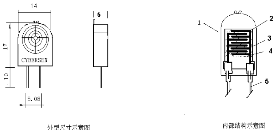
外型尺寸示意图
