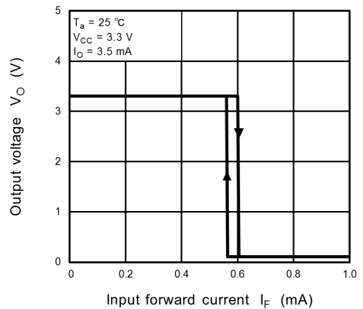
Fig. 12.2.12 V_O - I_F
