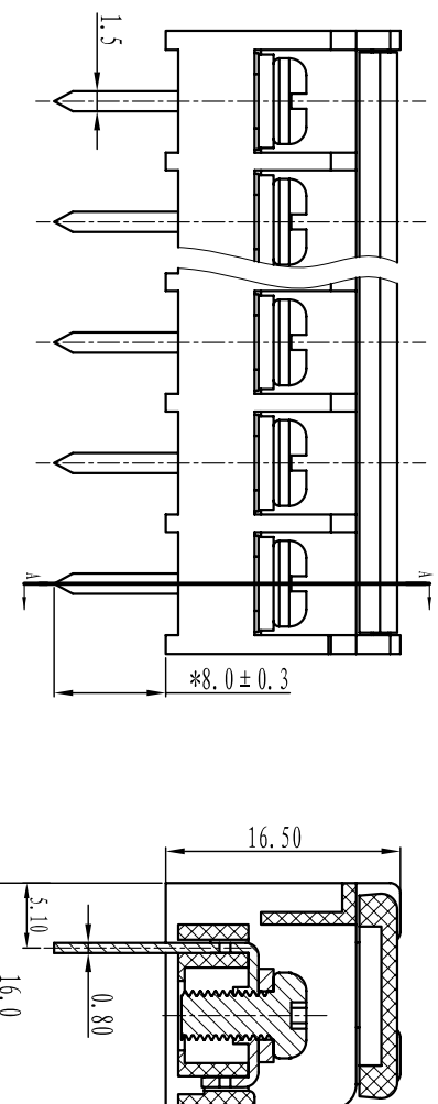
SECTION A-A
