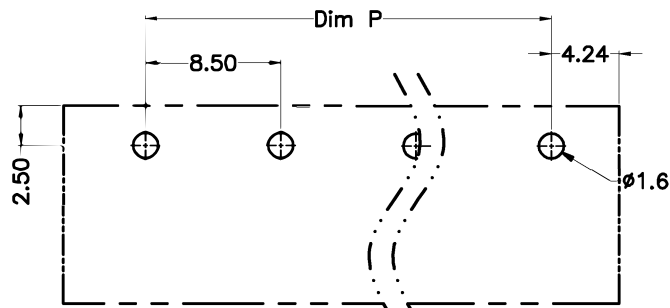
P.C.B.LAYUOT
