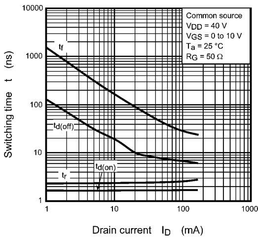
Fig. 7.9 t - I_D
