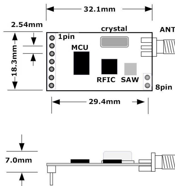
图一 产品尺寸图
