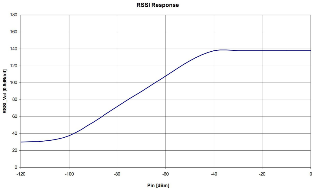
图五 场强动态范围
