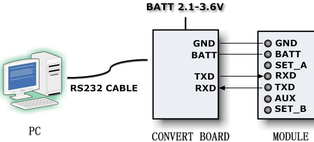
图七 软件设置接线图
