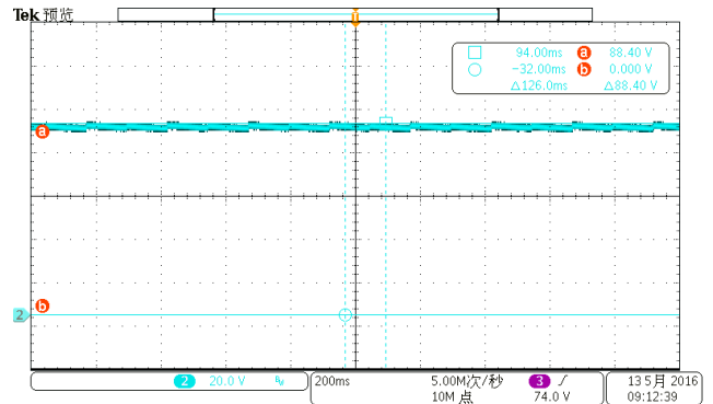
264Vac CH3:Vo
