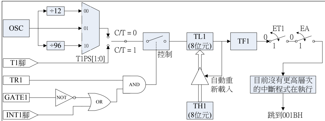
图 6-3: 模式 2 - 8 位自动重载定时/计数
