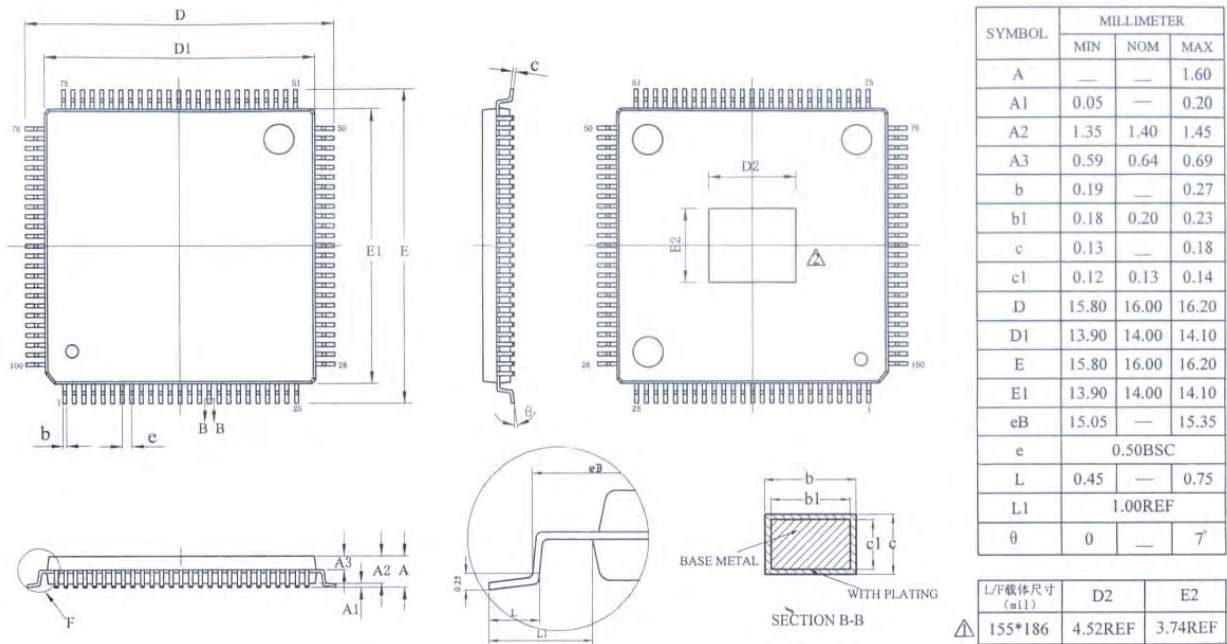
100 引脚裸露焊盘、超薄四方扁平封装[TQFP_EP](SV-100-4)尺寸(单位:mm)
