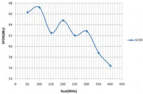
图 9 宽带 SFDR 与输出频率的关系
