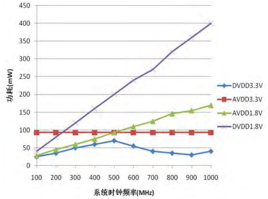
图 12 功耗与系统时钟的关系 (PLL 禁用)
