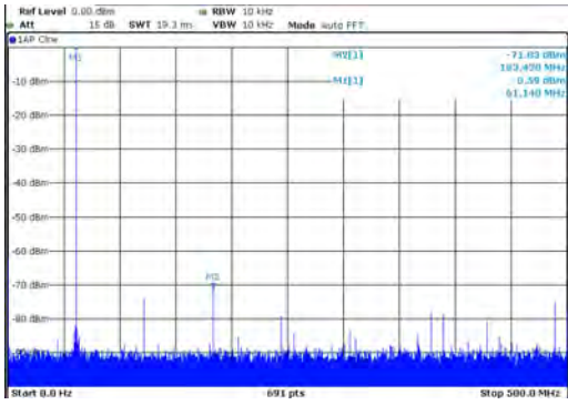
图 3 61.1MHz 条件下的宽带 SFDR, REFCLK=1GHZ
