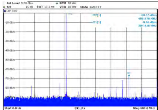
图 4 204.1MHz 条件下的宽带 SFDR, REFCLK=1GHZ
