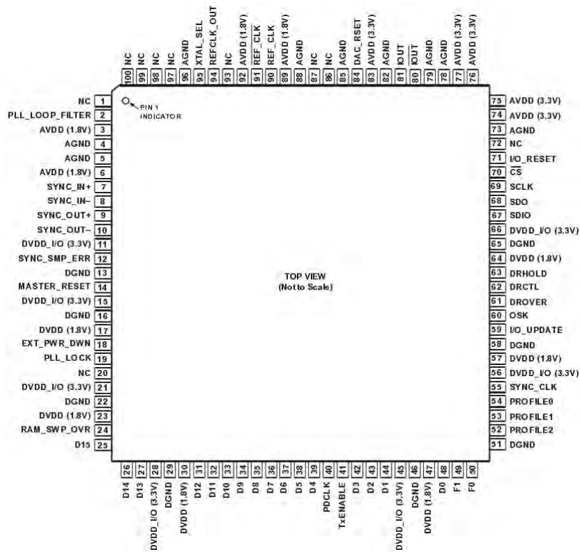
图 2 芯片管脚图
