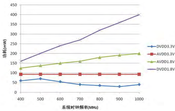
图 13 功耗与系统时钟的关系 (PLL 使能)
