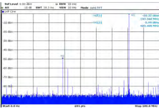
图 5 403.1MHz 条件下的宽带 SFDR, REFCLK=1GHZ
