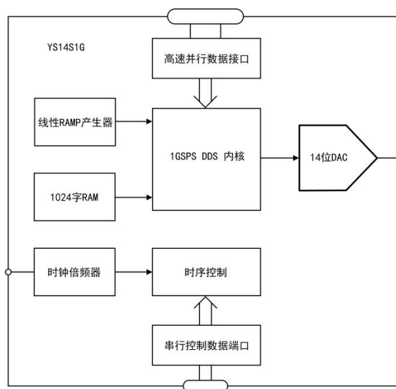
图 1 YS14S1G 功能框图
