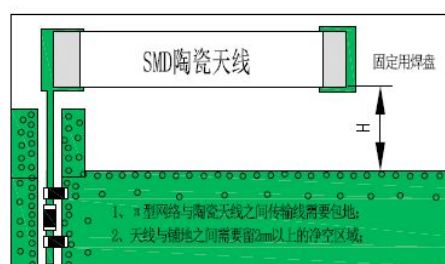
预留 π 型天线匹配网络
