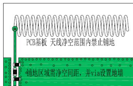
预留 π 型天线匹配网络
