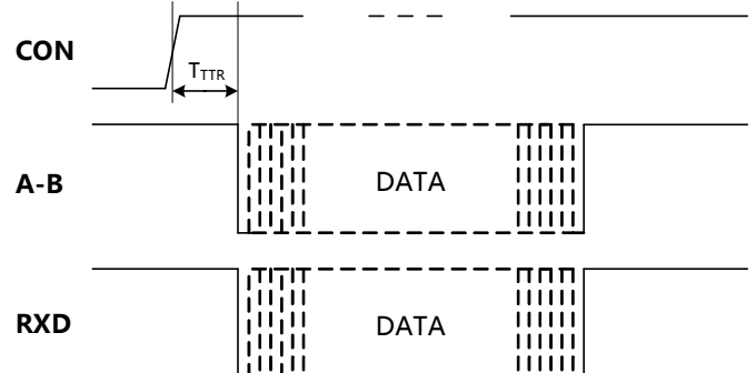
图 2. RSM(3)485CT模块数据接收时序图
