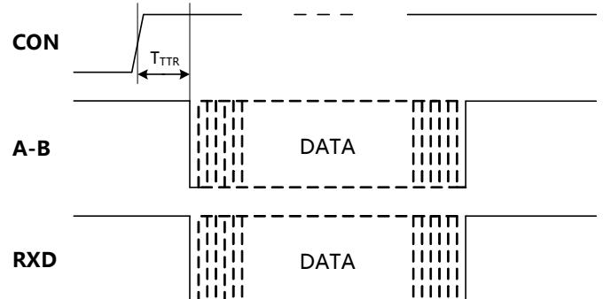
图 2. TDM(3)485CT模块数据接收时序图
